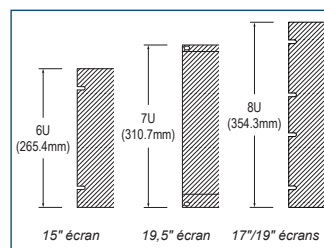
Hauteurs de panneau pour les écrans rackables de Hope Industrial Systems.
